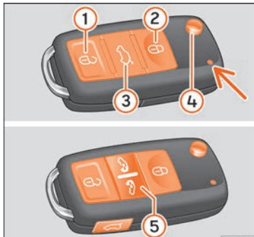
Abb. 86 Tasten im Funkschlüssel.
