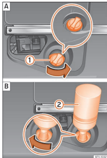
Abb. 284 AdBlue-Tank mit Verschluss des Tankeinfüllstutzens und Nachfüllflasche.
