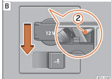
Abb. 70 Seitenbereich des Gepäcksraums: A Ausbau Rückleuchte links. B Ausbau Rückleuchte rechts.
