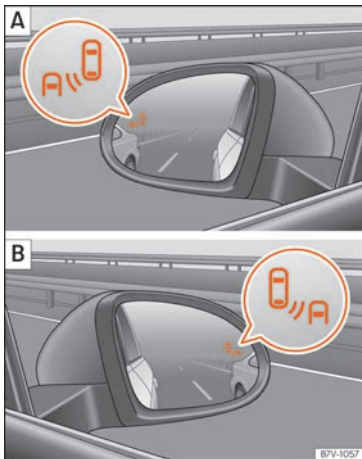
Abb. 262 An den Außenspiegel: Anzeige des Blind-Spot-Assistenten.
