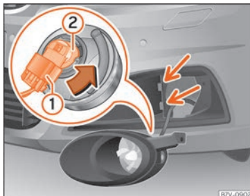
Abb. 67 Glühlampe im Scheinwerfer austauschen.
